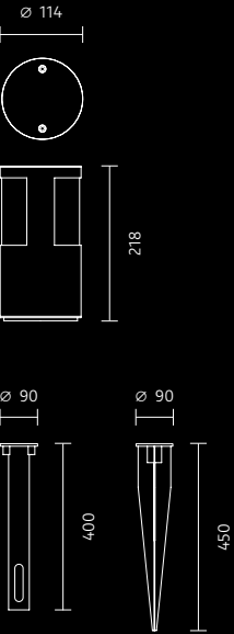
Erdanker und Erdspieß / Ground anchor and ground spike
