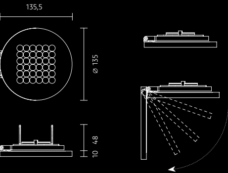
für Hohlraumeinbau / for cavity mounting
